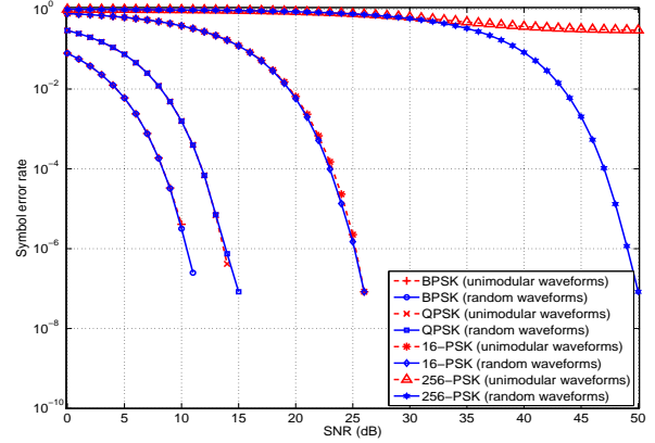
Fig. 3. SER versus SNR.
